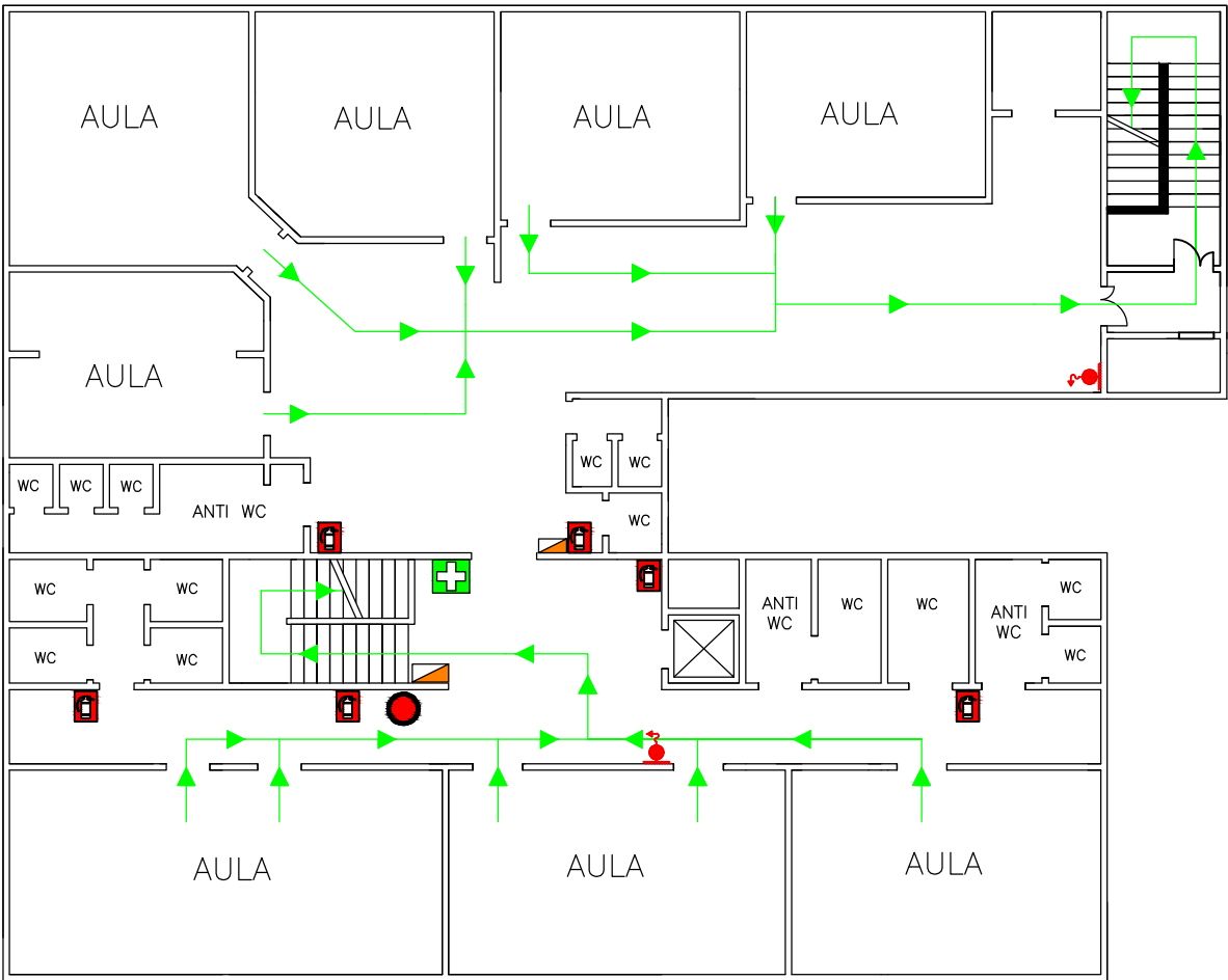
PIANO PRIMO
